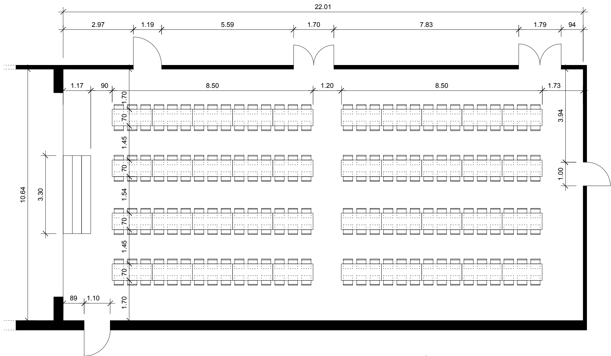
Gemeindesaal 8926 Kappel am Albis Bankettbestuhlung maximal 240 Personen 25.04.2010 1:100
